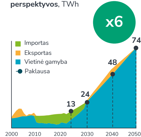
Lietuvos elektros energijos paklausos ir pasiūlos perspektyvos, TWh
